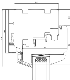
Oberer Türrahmen
