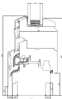
Bodenschwelle holz
