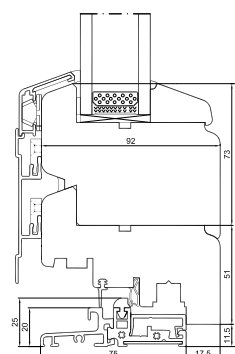
Bodenschwelle Aluminium
