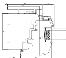
Seitenrahmen
