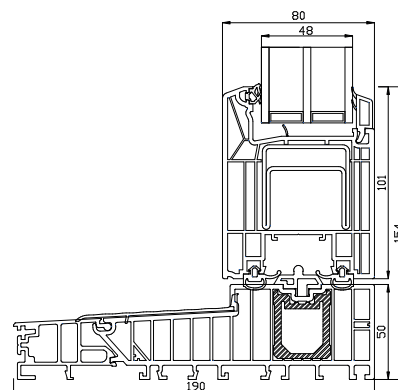
Türschwelle
