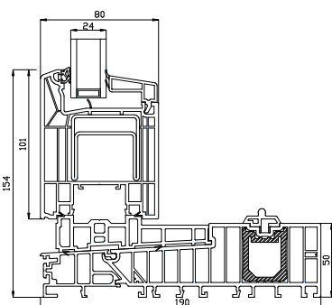
Türschwelle
