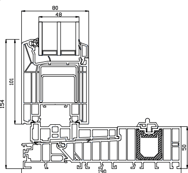
Türschwelle
