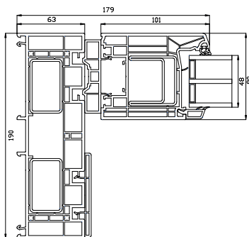
Seitenrahmen
