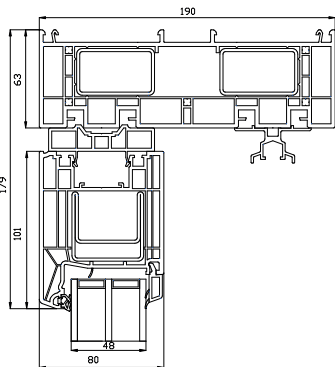
Oberer Fensterrahmen
