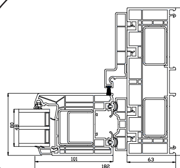
Seitenrahmen
