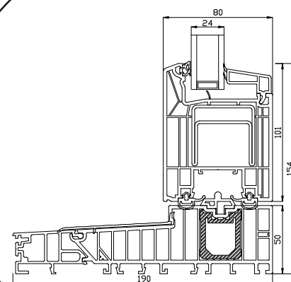
Türschwelle
