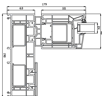
Seitenrahmen
