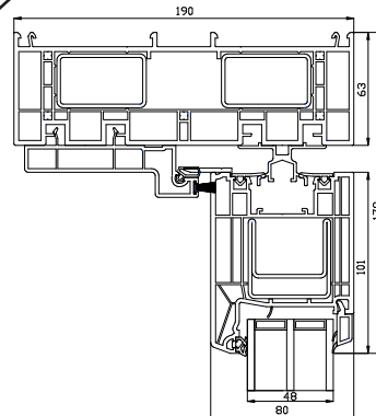
Oberer Fensterrahmen
