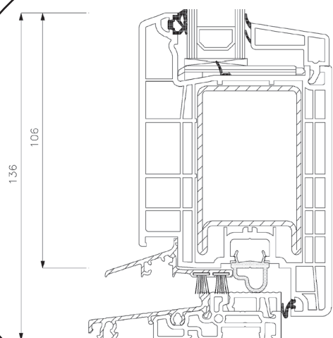
Türschwelle
