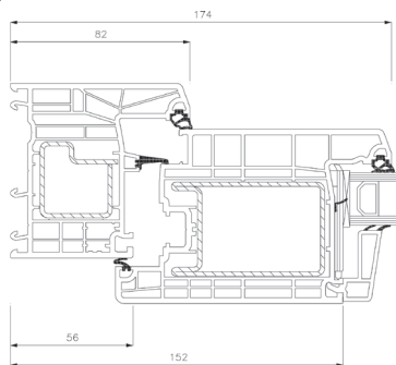
Seitenrahmen
