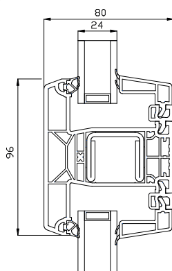
Querprofil
