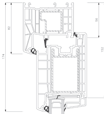
Oberer Türrahmen
