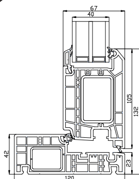
Türschwelle
