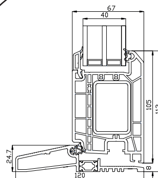
Bodenschwelle Aluminium
