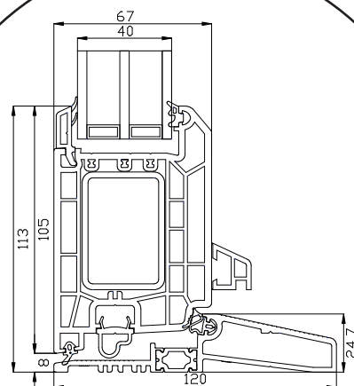
Türschwelle
