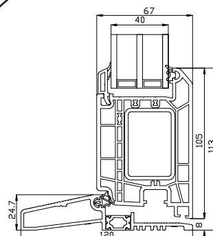
Bodenschwelle Aluminium
