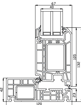
Türschwelle
