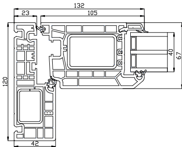
Seitenrahmen
