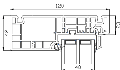
Oberer Türrahmen
