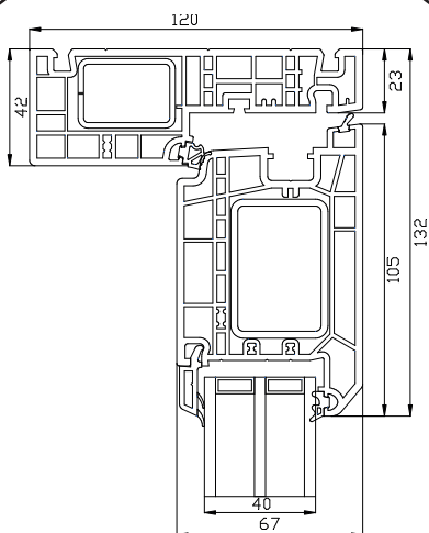
Oberer Türrahmen
