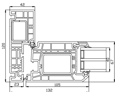
Seitenrahmen
