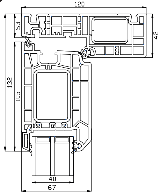
Oberer Türrahmen
