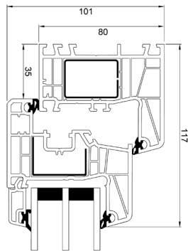
Oberer Türrahmen
