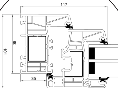
Seitenrahmen
