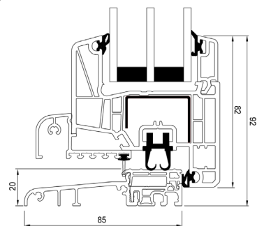
Niedrige Alu-türschwelle
