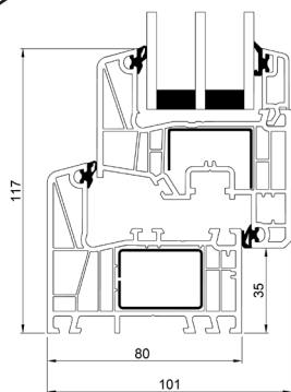
Bodenschwelle Kunststoff
