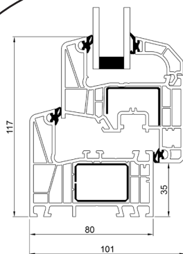
Bodenschwelle Kunststoff
