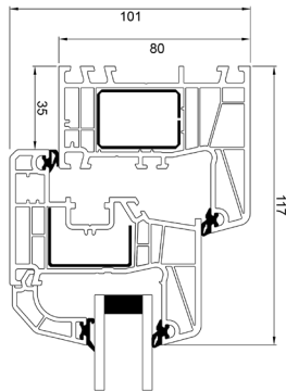
Oberer Türrahmen
