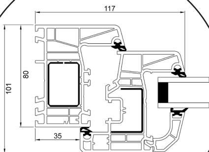
Seitenrahmen
