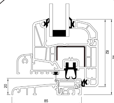
Niedrige Alu-türschwelle
